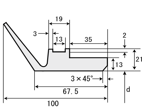
取付前の寸法
