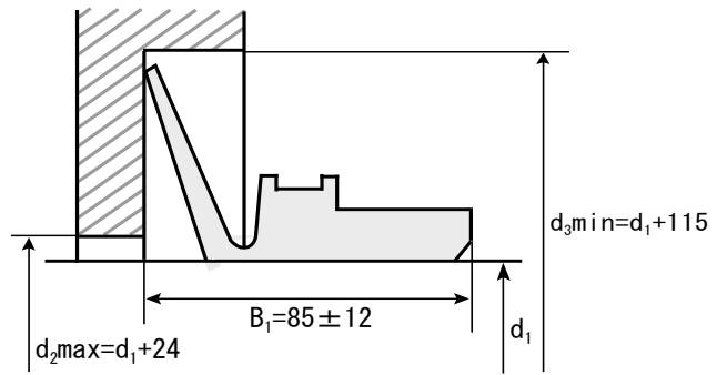
取付後の寸法
