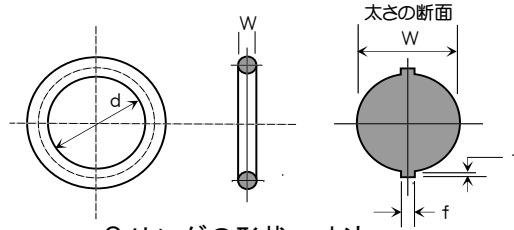
Oリングの形状・寸法
