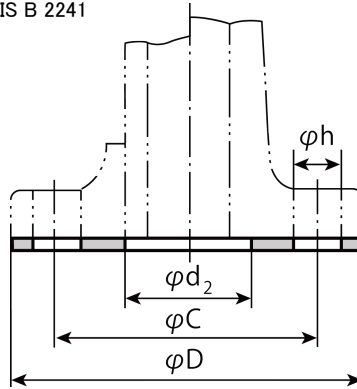
FF (非金属平形) ガスケットの形状・寸法
