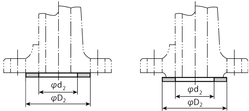
RF(非金属平形)ガスケットの形状・寸法
