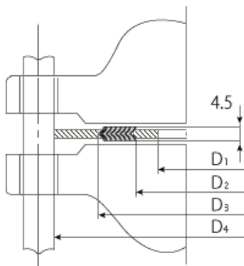
うず巻形ガスケット(内外輪付き)の形状・寸法
