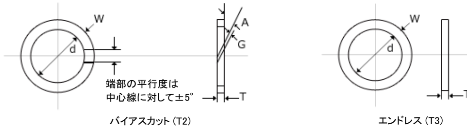
リングの形状・寸法
